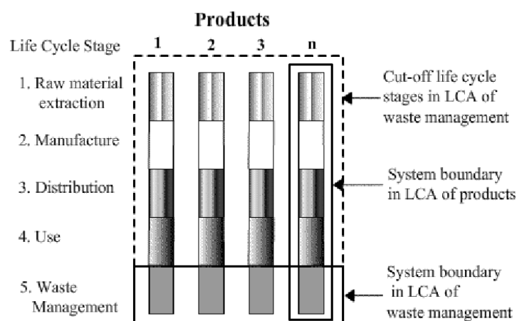
Figura 1. Diferències en l'abast del ACV de la gestió de residus i l'ACV de producte. Font: ResearchGate
