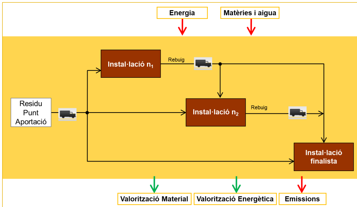
Figura 5 Límits del sistema d'estudi.
